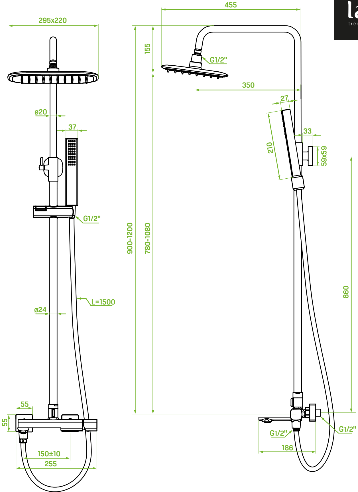
LAVEO - TORES PLT x0KB 1:7 (mm)
