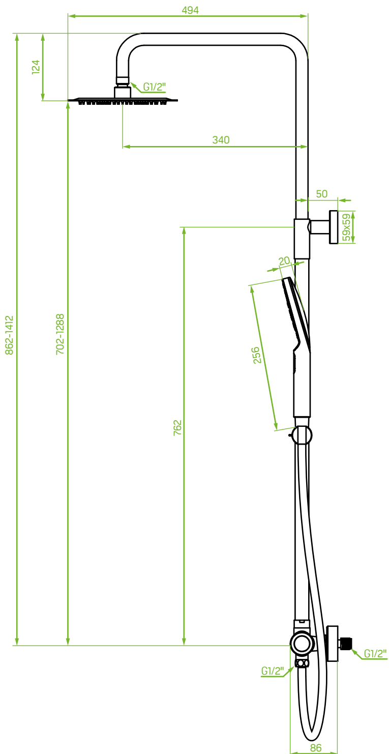
LAVEO - VOLUMO PLV x00B 1:7 (mm)
